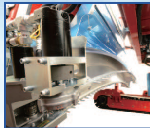
●2段刈摘採ユニット (中央搭載)
